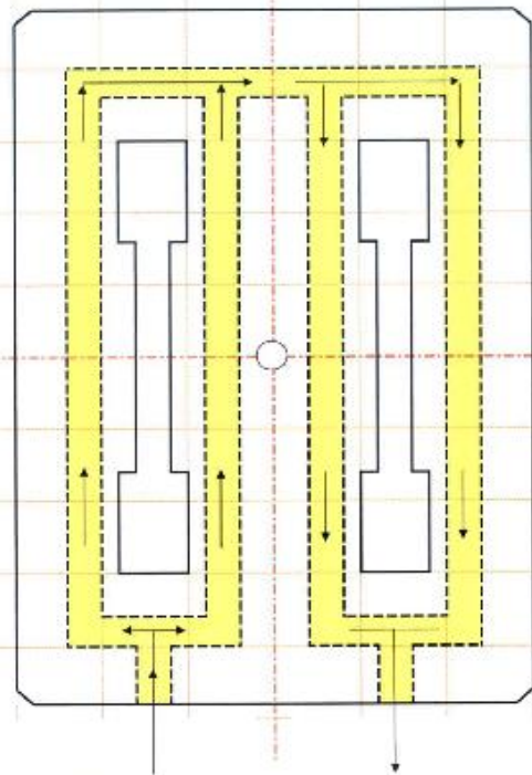
アキシコンタイプの温調回路図
